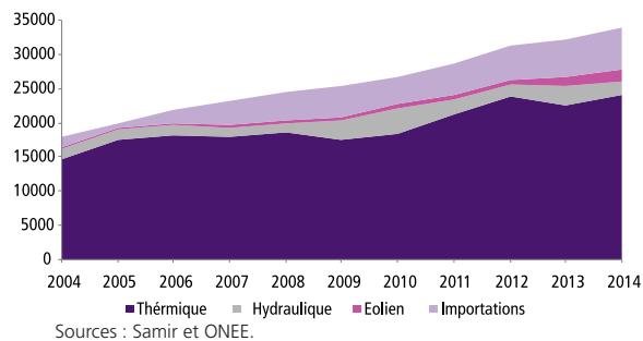
Graphique 1.2.6 : Structure de l'électricité disponible par source primaire (en GWh)
