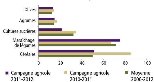
Graphique 1.2.3 : Principales productions végétales (en millions de quintaux)
