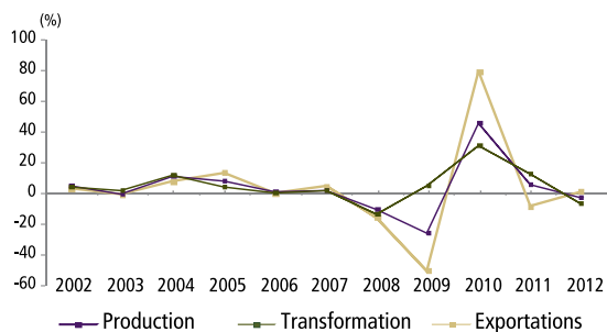
Graphique 1.2.8 : Variations de la production et des utilisations de phosphate brut en volume
